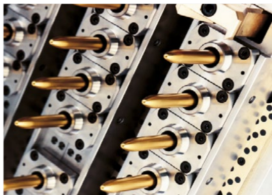
Abbildung: Auswerferstifte
